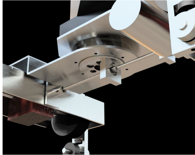
Eine besondere Herausforderung stellte der Allrad-Antrieb unter Berücksichtigung der Gelenke dar. (Rendering)
